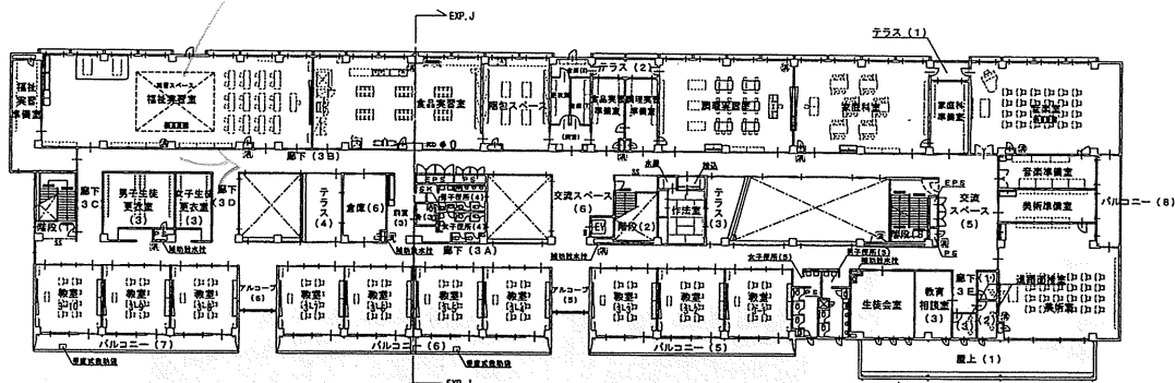
【 3 階 平面図 】
