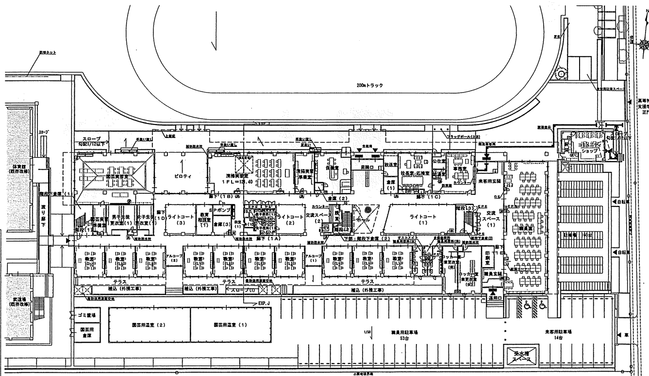
【 2 階 平面図 】
